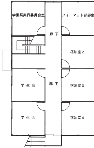
2階 平面図
